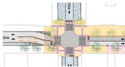
Návrh úprav křižovatky Pernerova × Kollárova
